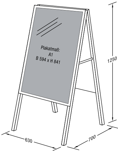
T-AS 1 mit 2 Wechselrahmen
