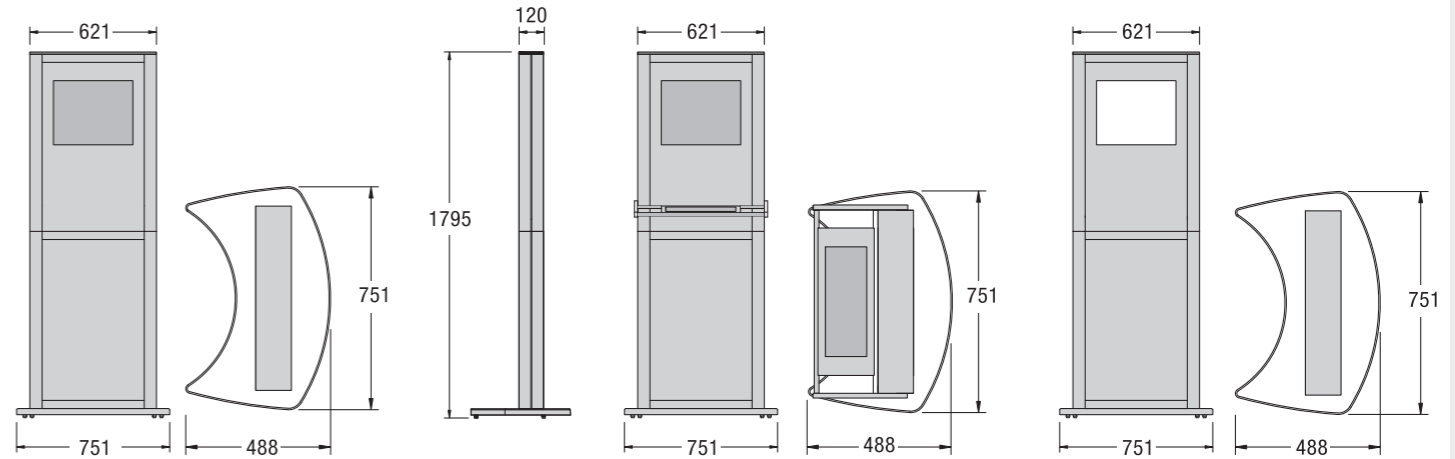
OT 10 OCTAterminal mit 19"- Monitor, ohne Tastatur, ohne Rechner
