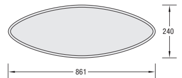
VA 7501 Abdeckplatte für VA 7500 Holz, 10 mm, schwarz
