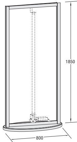
VA 7500 Grund-Set Säule Sockel, Holz schwarz, Lieferumfang ohne Panels
